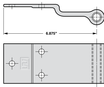
Side Door Hinge Strap
