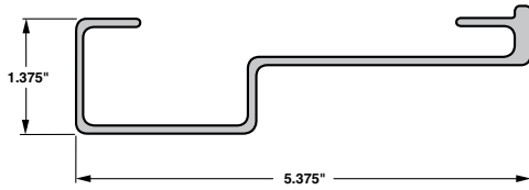
Side Door Post H/S
